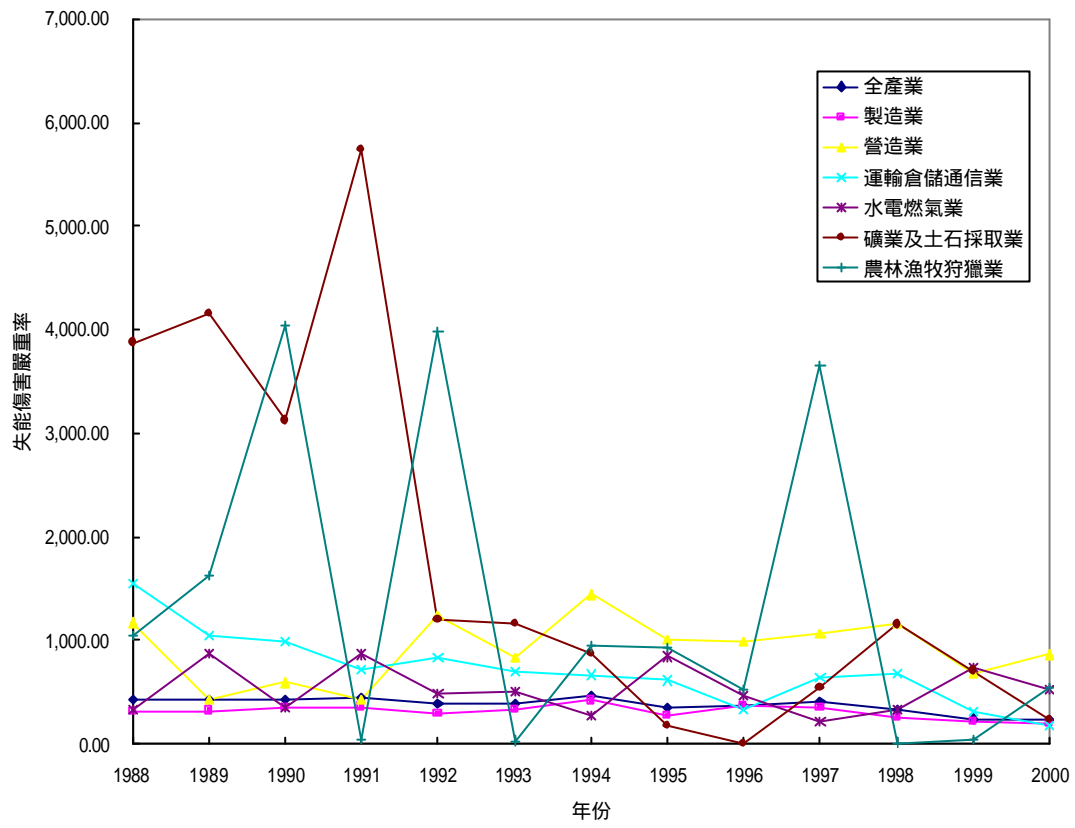
圖 2-1 1988- 2000 年職業災害統計概況—失能傷害嚴重率
